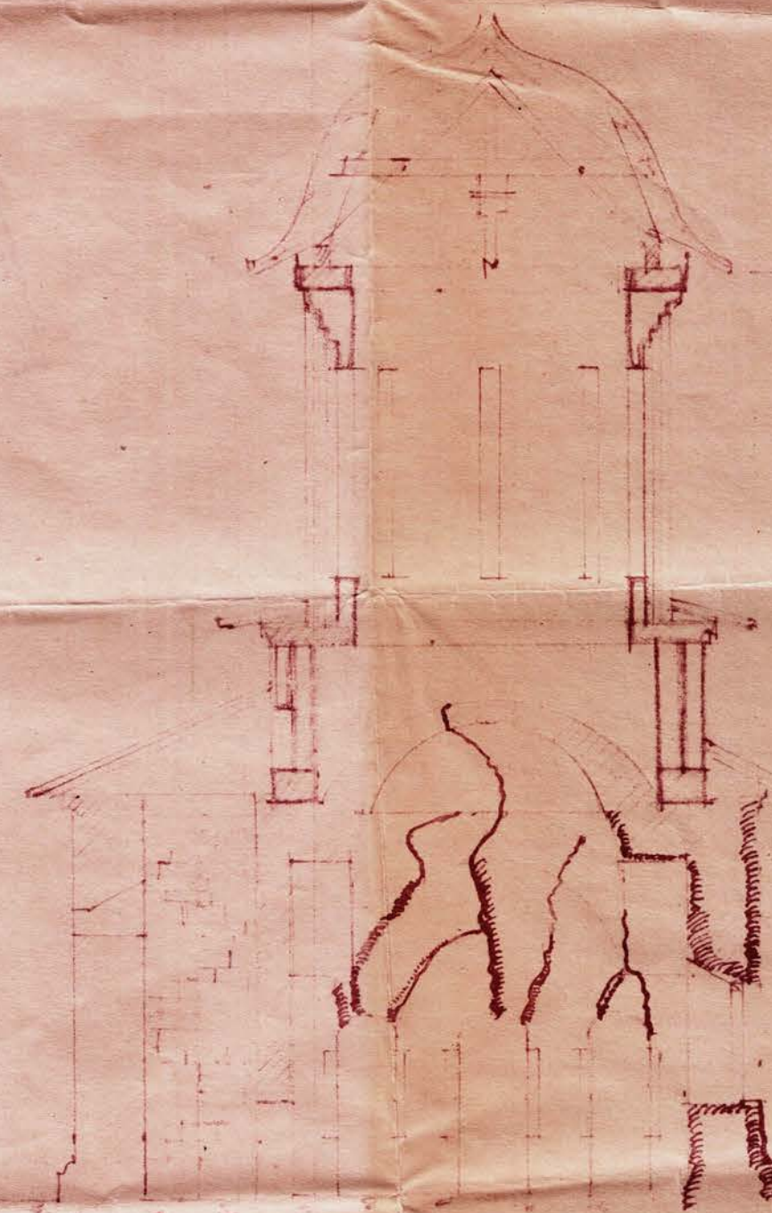
SECȚIE TRANSVERSALĂ PRIN BISERICA ȘI TURLE. SECT. CIRCULĂTORIE
