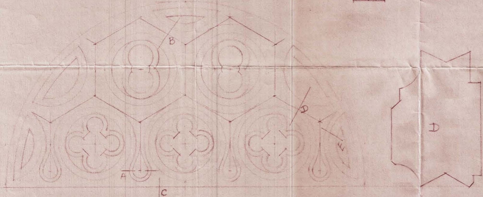
DETALIUL TIMPANULUI SCARA 0M20 = 1METRU
