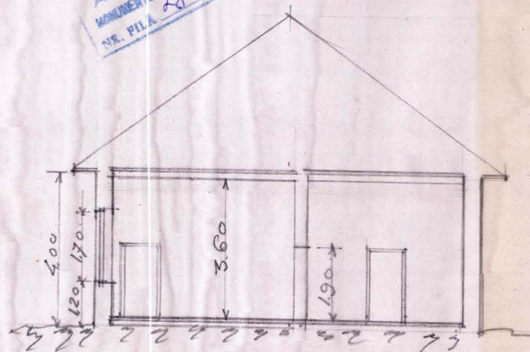
=SECTIE TRANSVERSALA=
