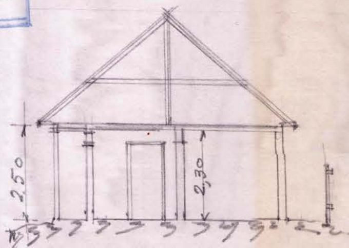
— SECȚIE TRANSVERSALĂ —
